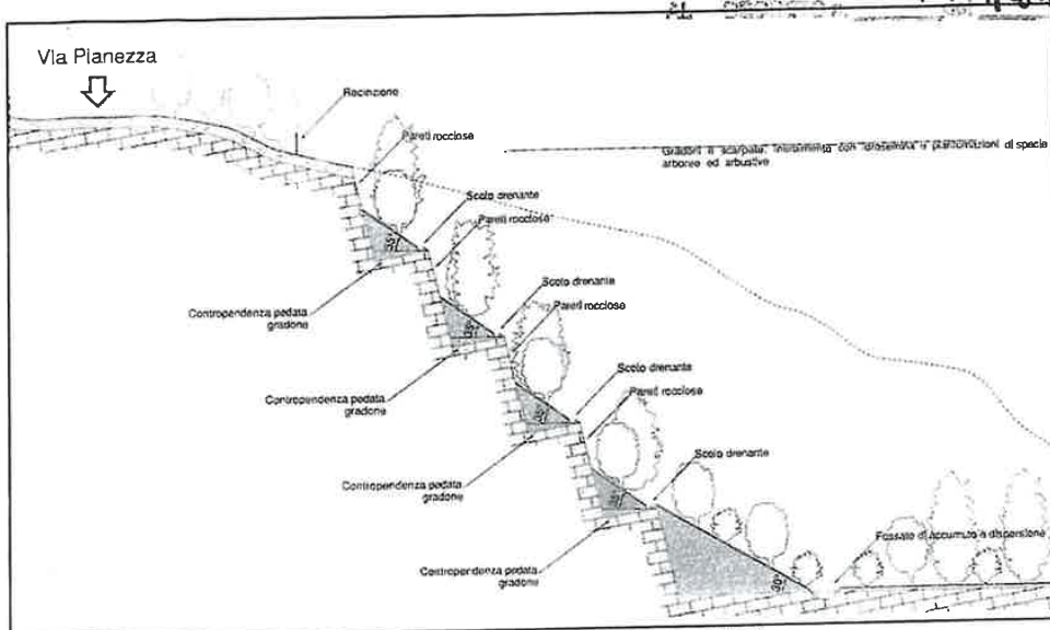
Sezione tipo - ricomposizione dei gradoni
