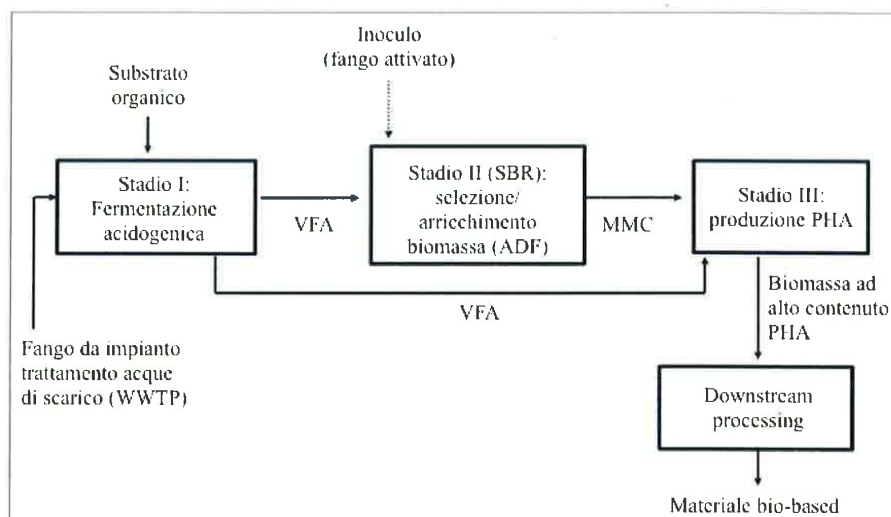
Figura 1 - Schema di processo a tre stadi maggiormente applicato per la produzione di PHA da MMC
