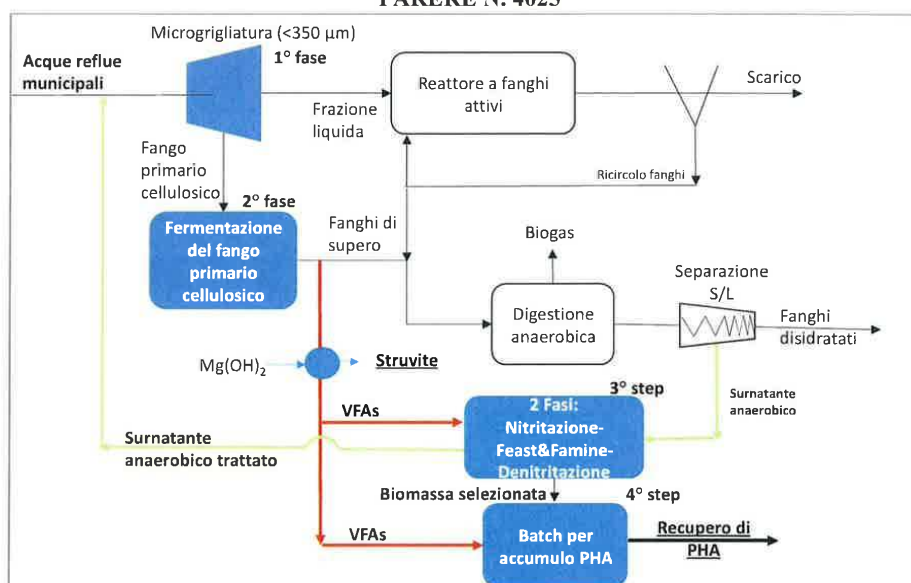
Figura 2 - SCEPPHAR integrato nella linea di trattamento fanghi (Azione Horizon2020 "SMART-Plant")
