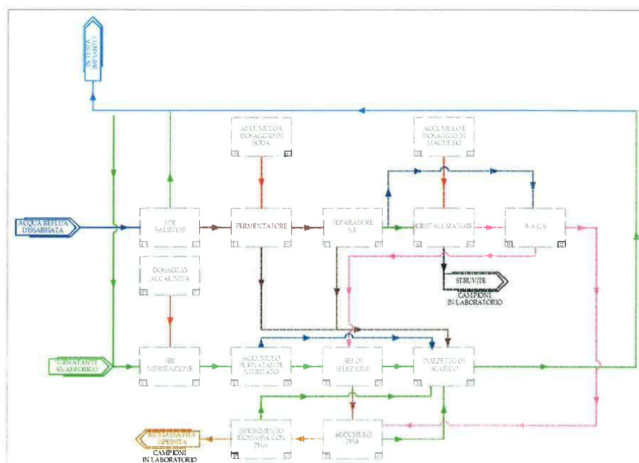
Figura 3 – Schema a blocchi del Sistema SCEPPHAR
