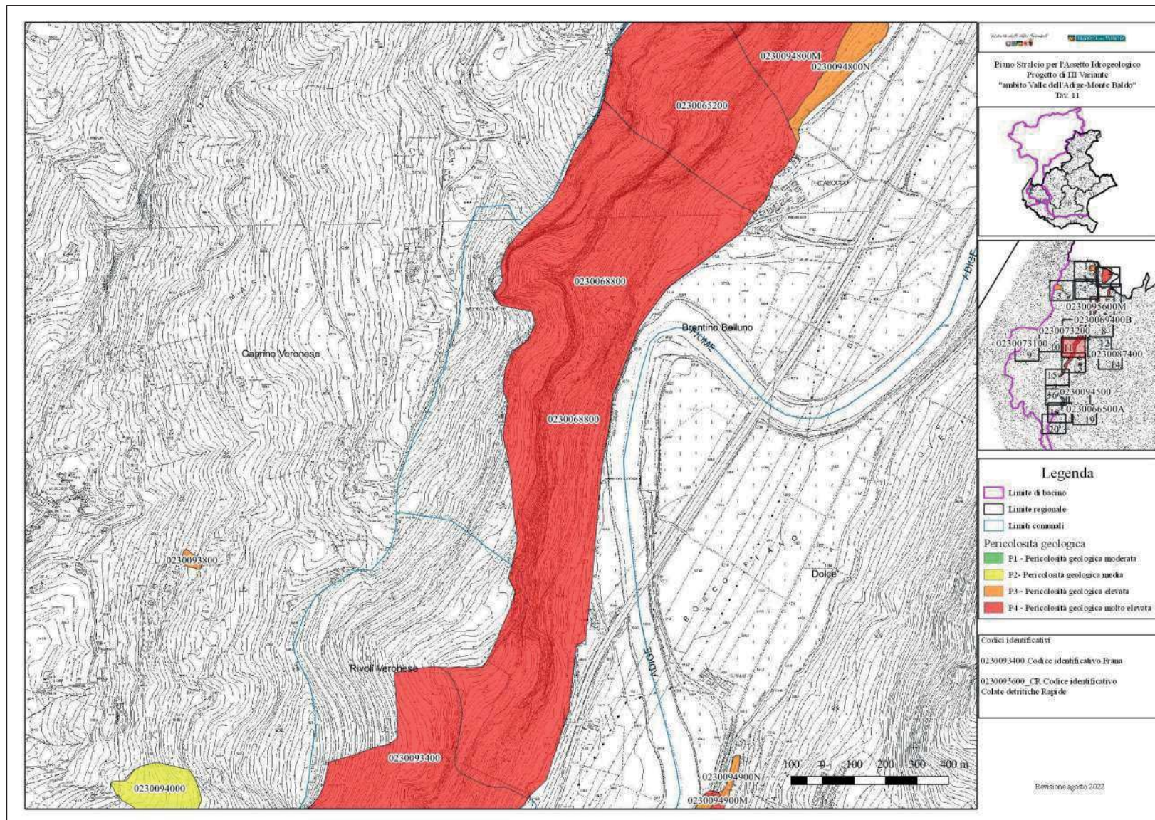
Tav. 11 – Carta della pericolosità geologica - Brentino Belluno, Caprino Veronese, Dolce e Rivoli Veronese.
