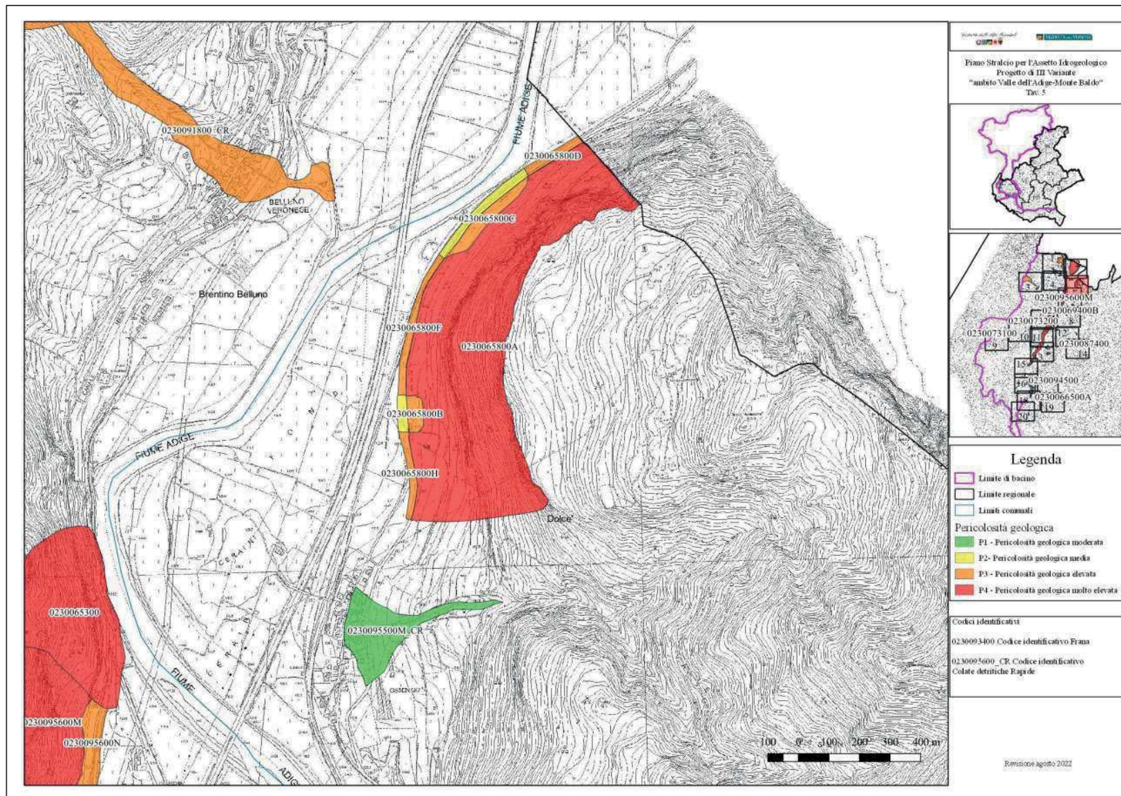
Tav. 5- Carta della pericolosità geologica - Brentino Belluno e Dolce.
