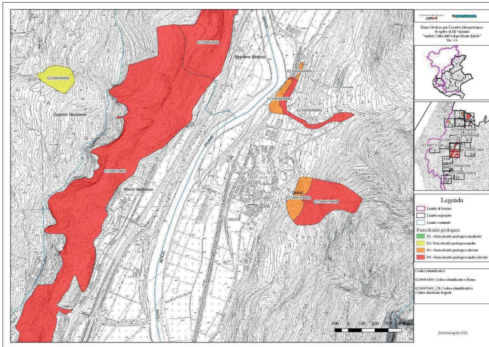
Tav. 13 – Carta della pericolosità geologica - Brentino Belluno, Caprino Veronese, Dolce e Rivoli Veronese.
