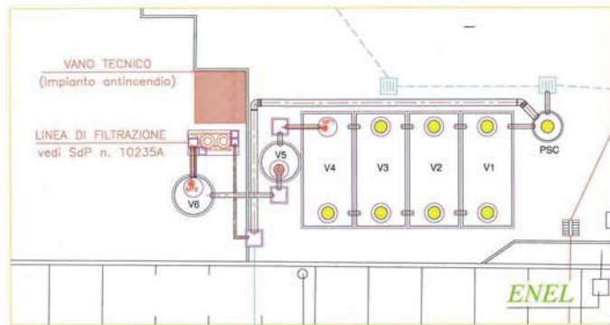
PARTICOLARE SCARICO S2 scala 1:100
