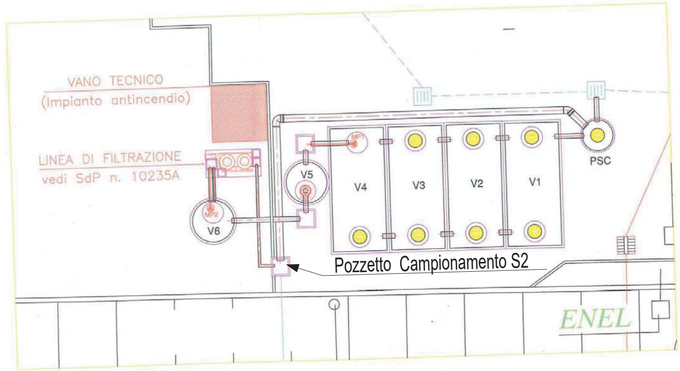
PARTICOLARE SCARICO S2 scala 1:100
