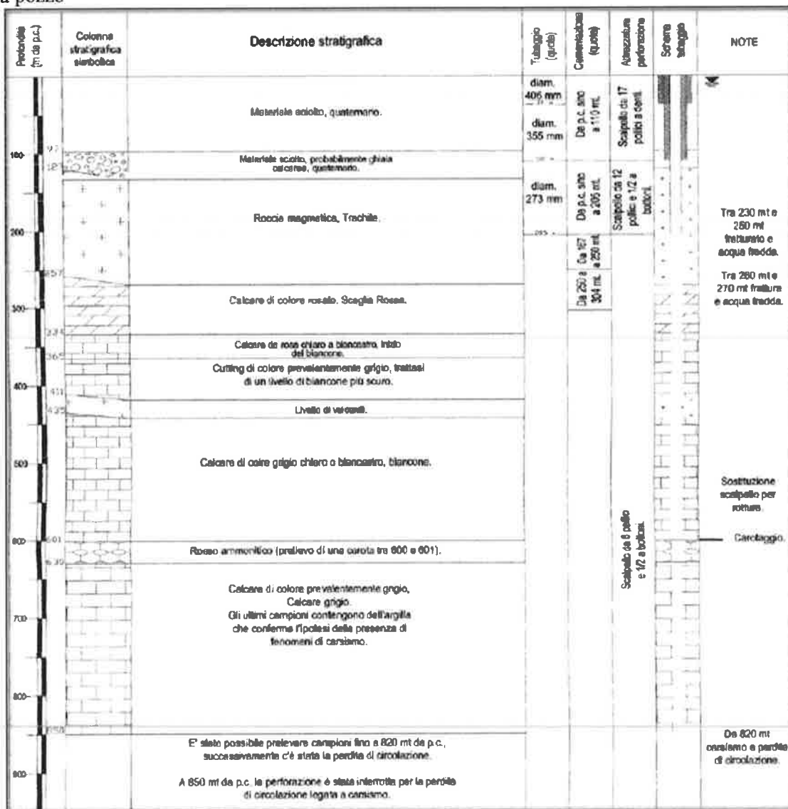
Schema pozzo
