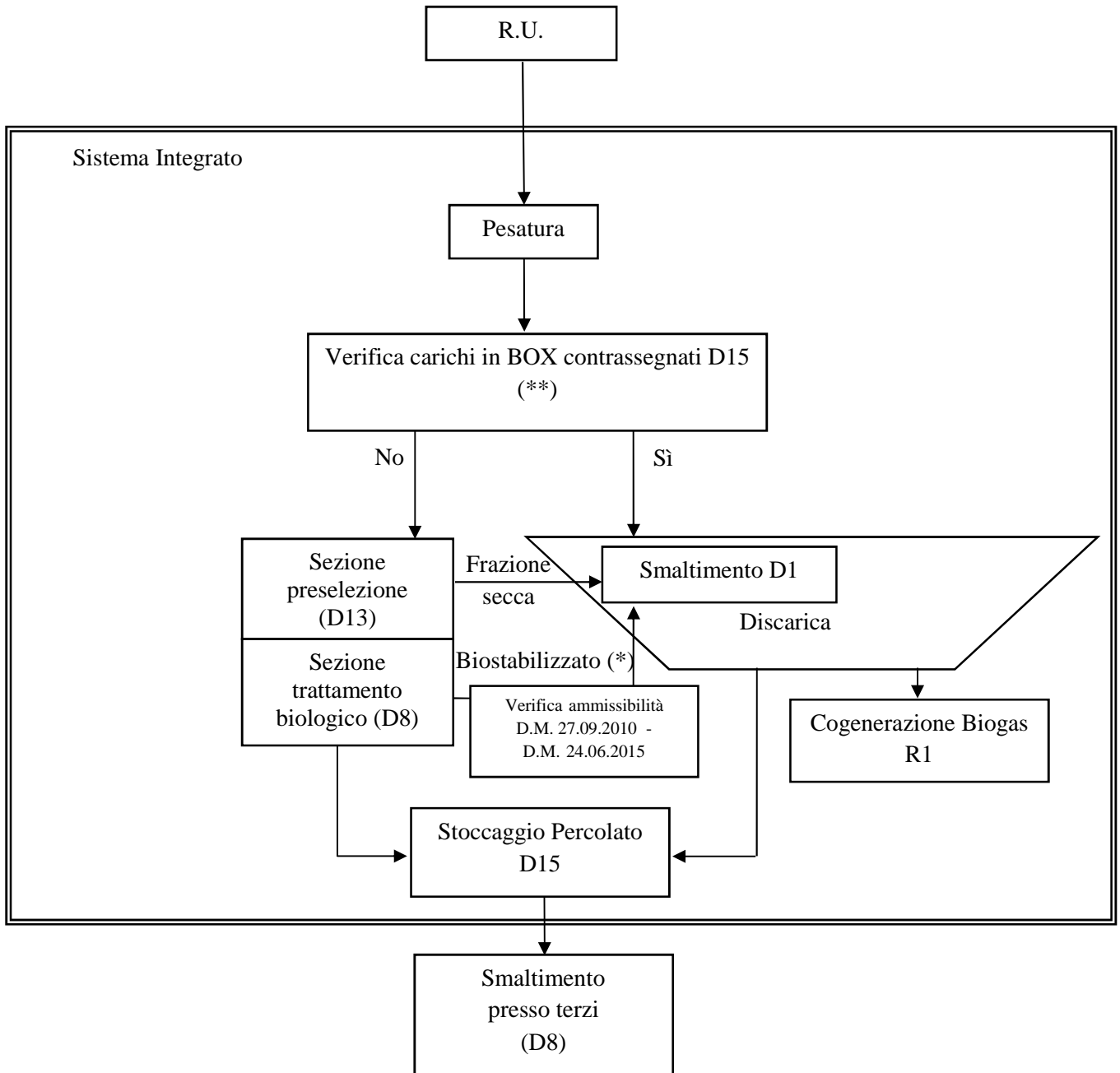
Schema A6.1 - (R.U. Avviati a smaltimento)
